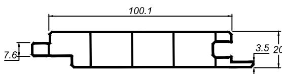
2072 PAINEL 100 X 20
