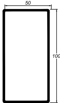
REF2003 (e=2mm)
