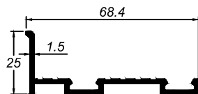
ALU4605 BASE DO TRILHO (68,4 x 25 x 1,5mm)
