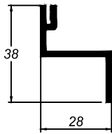
2070 PERFIL Z
