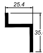
ALU2070 ACABAMENTO PISO - PORTA (25,4 x 35,6 x 2,6mm)
