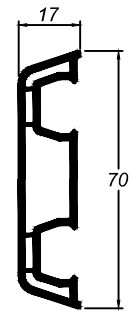
2036 GUARNIÇÃO 70
