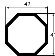
ALU2083 EIXO OCTOGONAL PERSIANA 40 mm (41 x 41 x 2mm)
